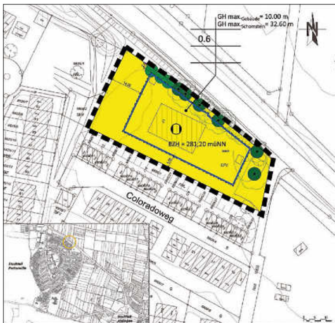
Bebauungsplan Lageplan
